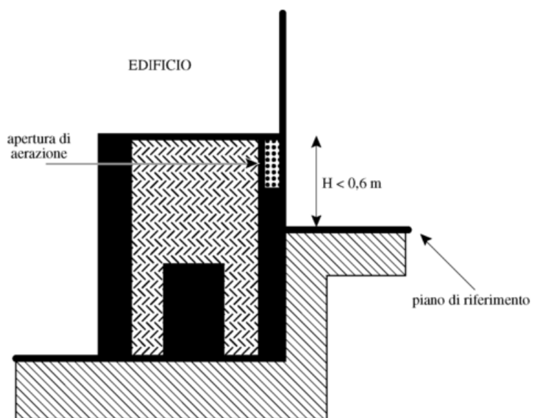
Tavola 3 - Locale seminterrato
