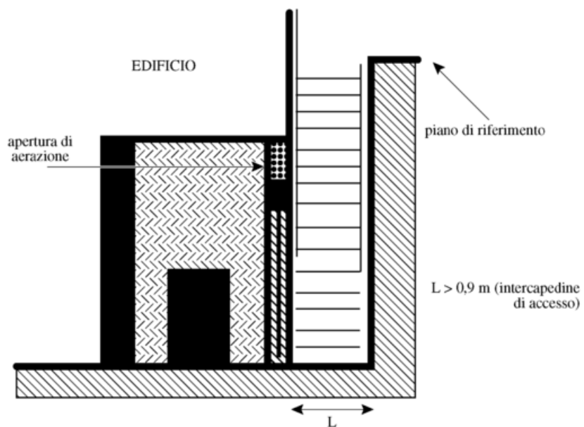
Tavola 2c - Locale interrato
