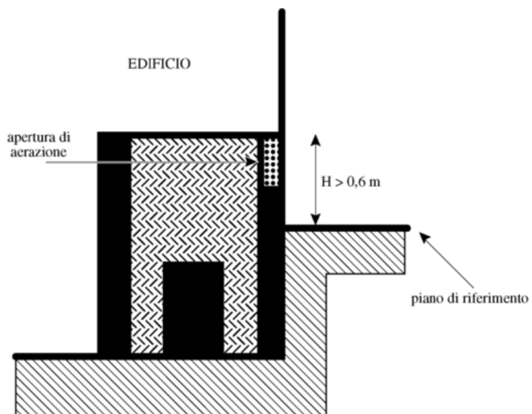
Tavola 4 - Installazione all'aperto in adiacenza a parete
