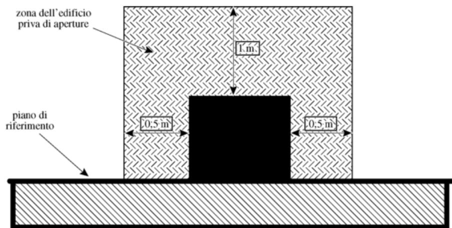
Tavola 4 - Installazione all'aperto in adiacenza a parete
